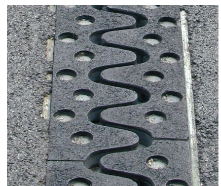
mageba RSFD Kragfingerfuge mit ROBO®GRIP
