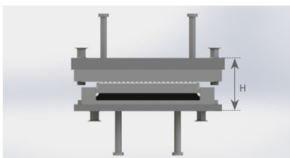
Schnitt durch TA Lager mit Ankerplatten mit Gewindehülsen
