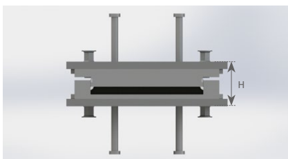
Schnitt durch TF Lager mit Ankerplatte mit Dollen
