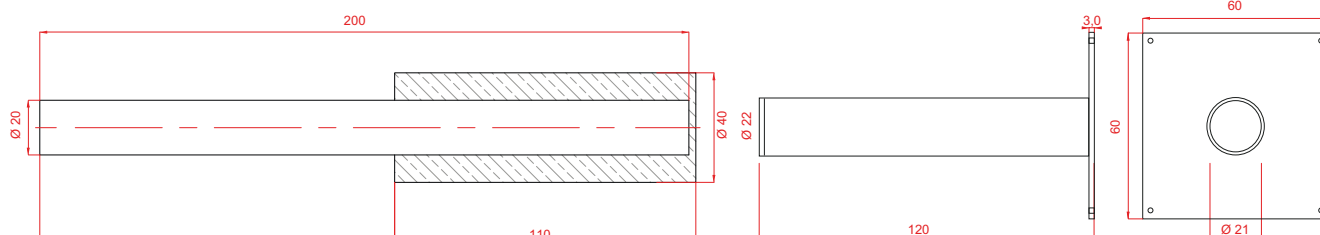
Sicherungsstift
