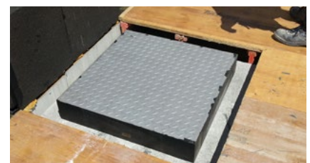
网纹钢板面的LASTO-BLOCK变形支座样例
