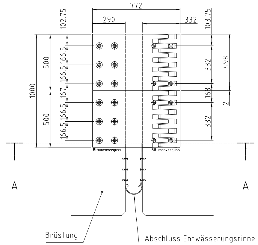
Draufsicht
