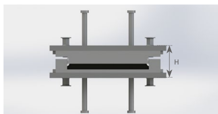
Sección de un apoyo TF con pernos (sin placas de anclaje)
