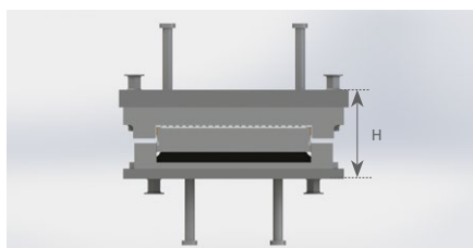
Sección de un apoyo TE con pernos (sin placas de anclaje)
