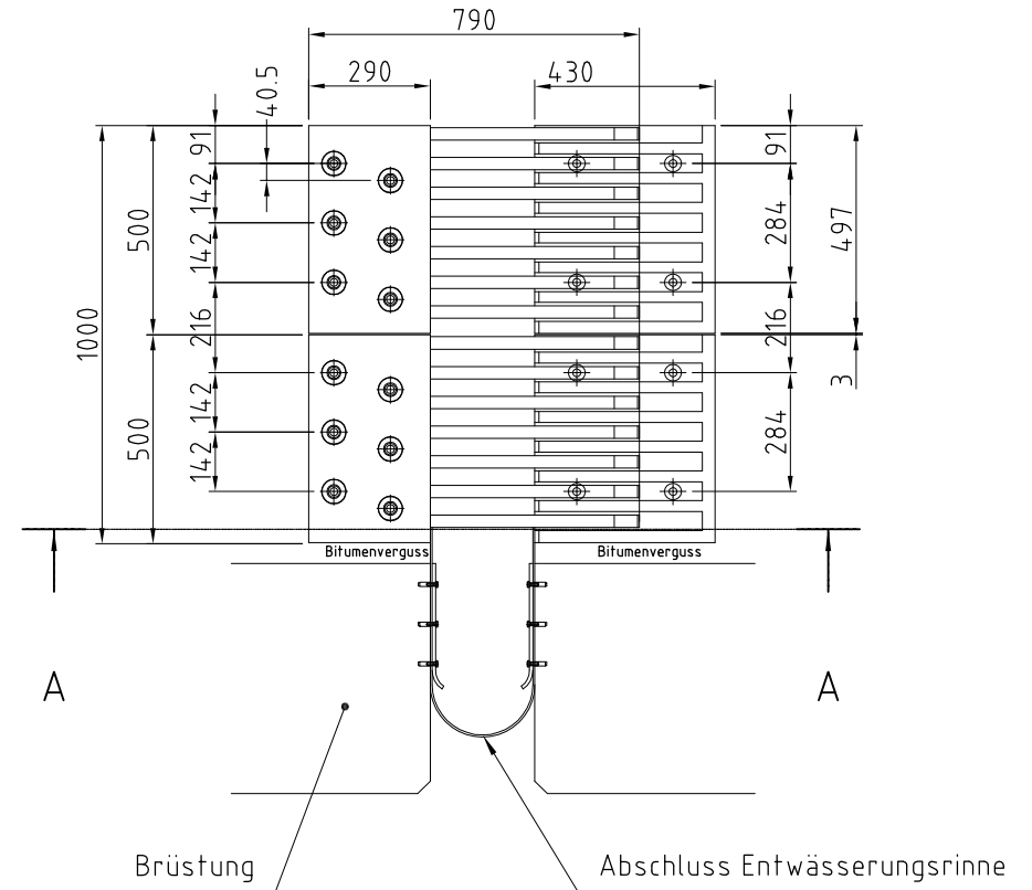
Draufsicht
