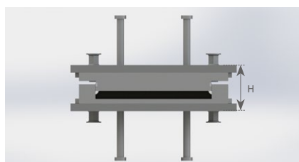
A TF típus keresztmetszeti képe horgonyzólemezek nélkül dübelekkel.
