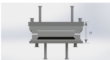
A TE típus keresztmetszeti képe horgonyzólemezek nélkül dübelekkel.
