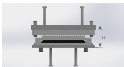
A TA típus keresztmetszeti képe horgonyzólemezek nélkül dűbelekkel.
