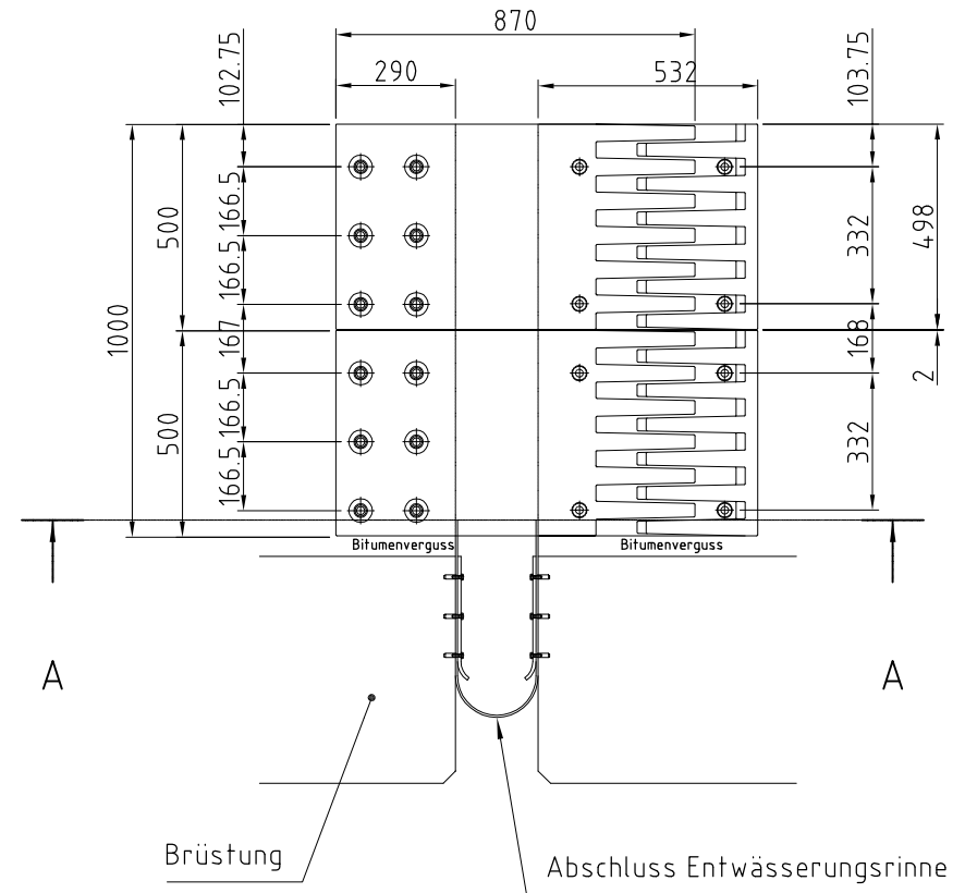
Draufsicht
