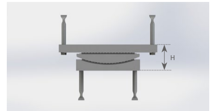
Ankraj plakasız, dişli manşonlu KA mesnetinin kesiti
