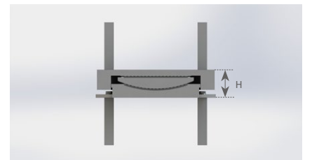
Ankraj plakasız, tespit pimli KF mesnetinin kesiti
