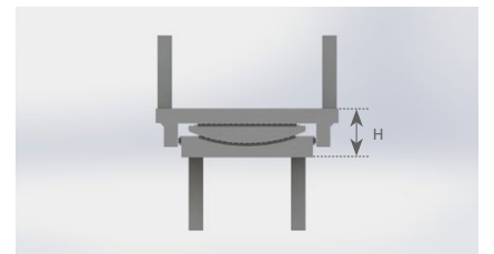
Ankraj plakası, tespit pimli KE mesnetinin kesiti
